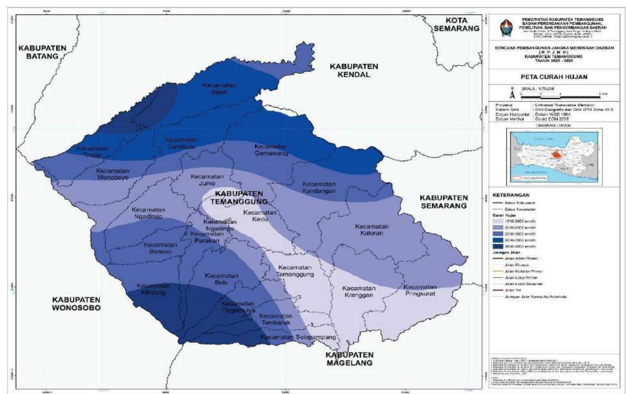
Gambar 2.5 Peta Curah Hujan Kabupaten Temanggung
